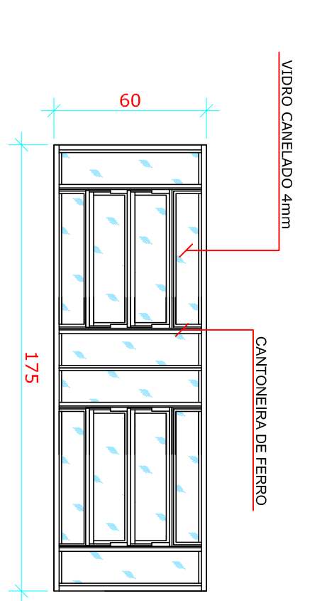
JB5 - JANELA BASCULANTE 175x60cm
