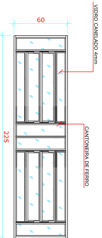
JB4 - JANELA BASCULANTE 225x60cm
