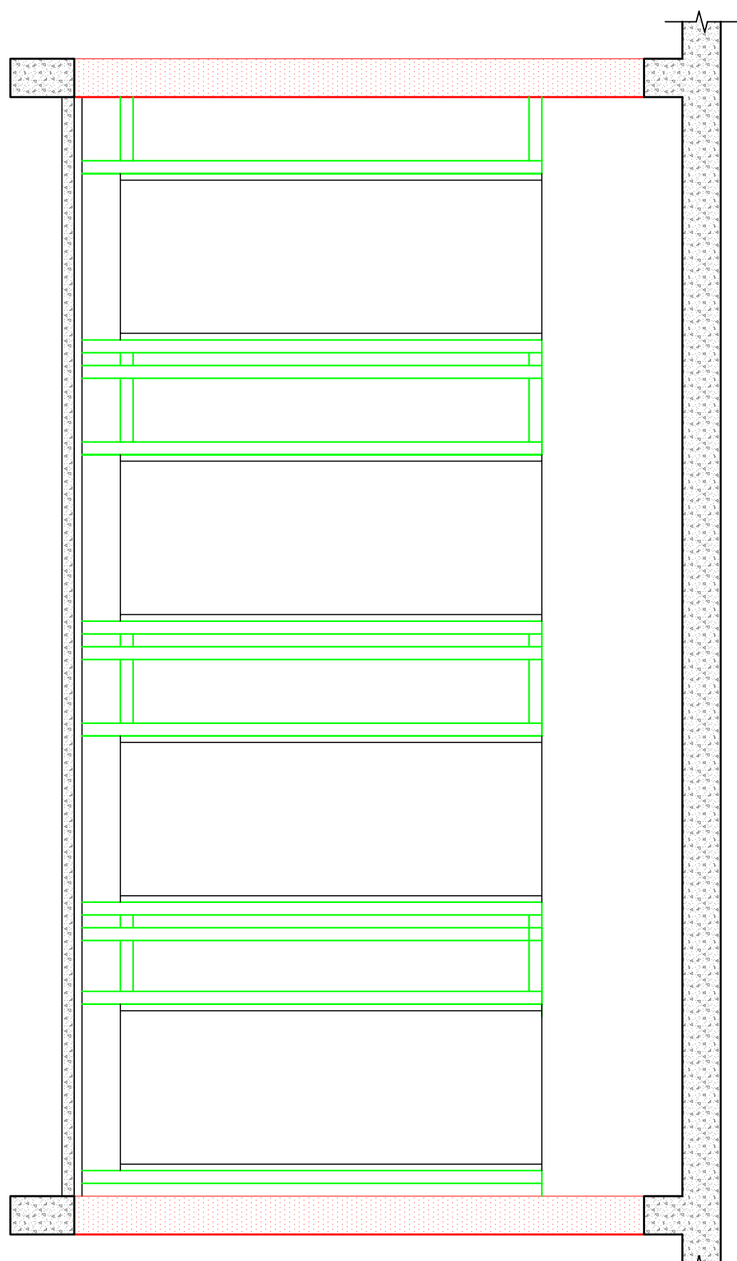
DETALHAMENTO DIVISÓRIAS DE EUCATEX
