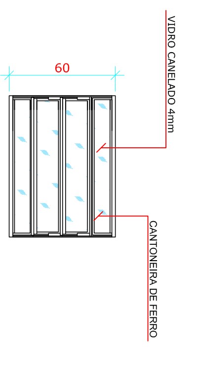
JJB5 - JANELA BASCULANTE 80X60cm
